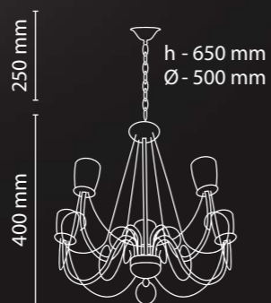
Vesta 10 340 8M-5 5×E14×60W 500×500×500 (0.125 m³)
