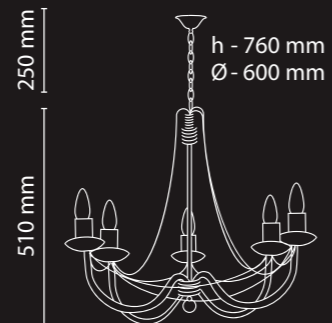
Vesta 12 340 N-5 5×E14×60W 600×600×520 (0.188 m³)
