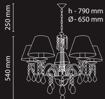
Grant 15 340CH 2SH-5 5×E14×60W 500×500×500 (0.125 m³)
